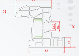
Pencere Kanat
