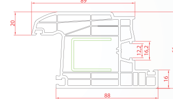
Kapı Kanat
