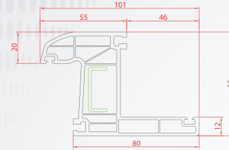
Pervazlı Kasa
